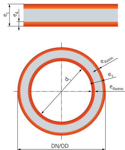
Przekrój rury strukturalnej z PVC-U typu A1
