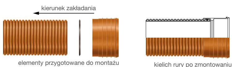
Fazy montażu kielicha
