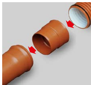
Zastosowanie łącznika do PVC
