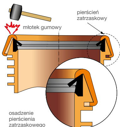
Uzbrajanie kielicha w uszczelkę
