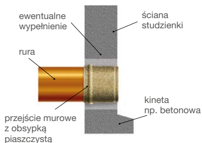
Typowe przejście rurociągu przez ścianę betonową
