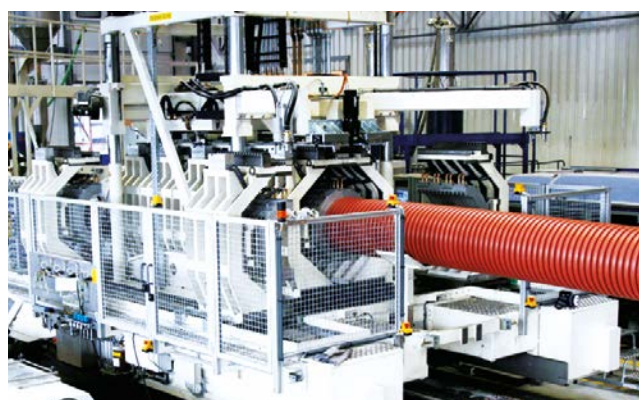
Proces formowania rur strukturalnych Pipelife.
