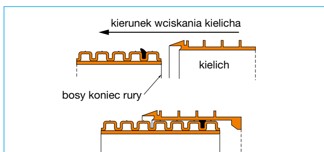
Schemat ideowy osadzenie uszczelki
